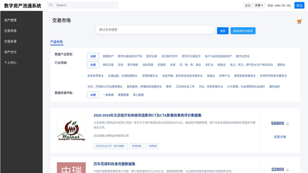
图 3-1 系统主界面整体布局（以交易市场页面为例）
