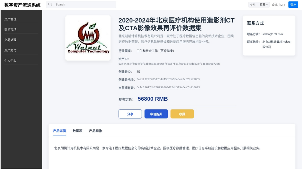
图 5-3 资产详情页面
