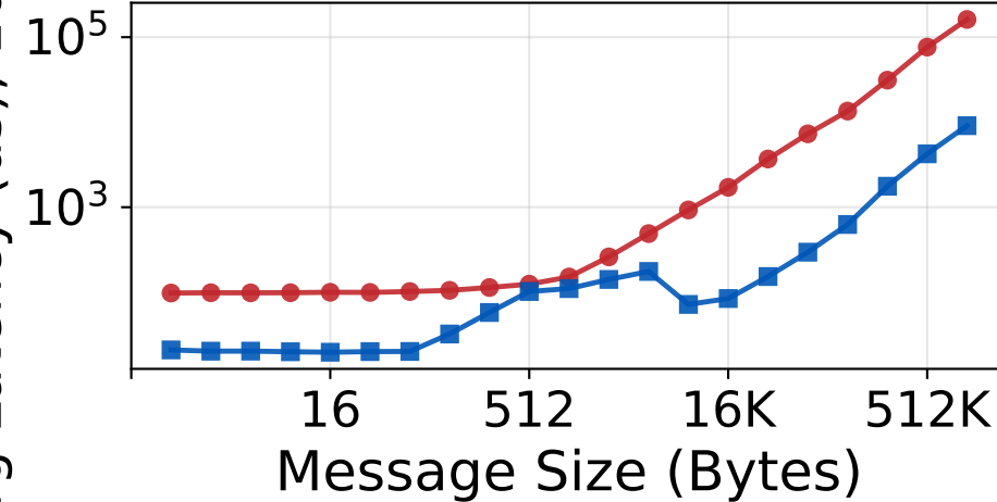
Allgather
