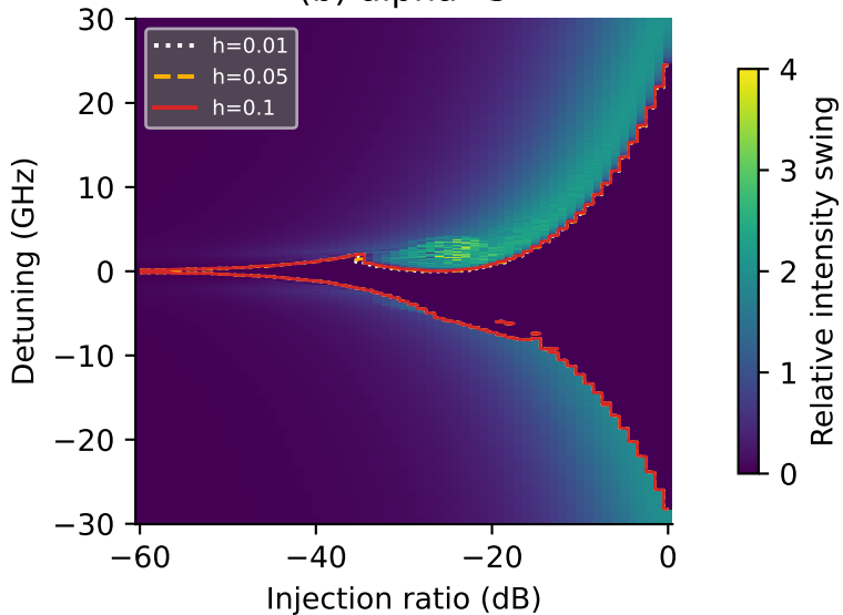
(b) \alpha=5
