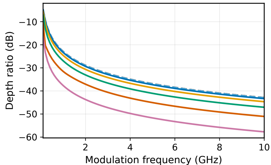
(d) PM-PM, \alpha = 5
