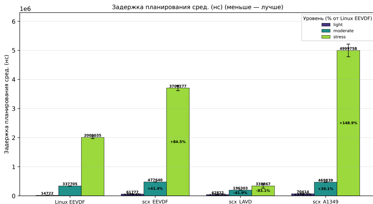
Рис. 5.1: Средняя задержка планирования (нс) для четырёх планировщиков по трём режимам нагрузки
