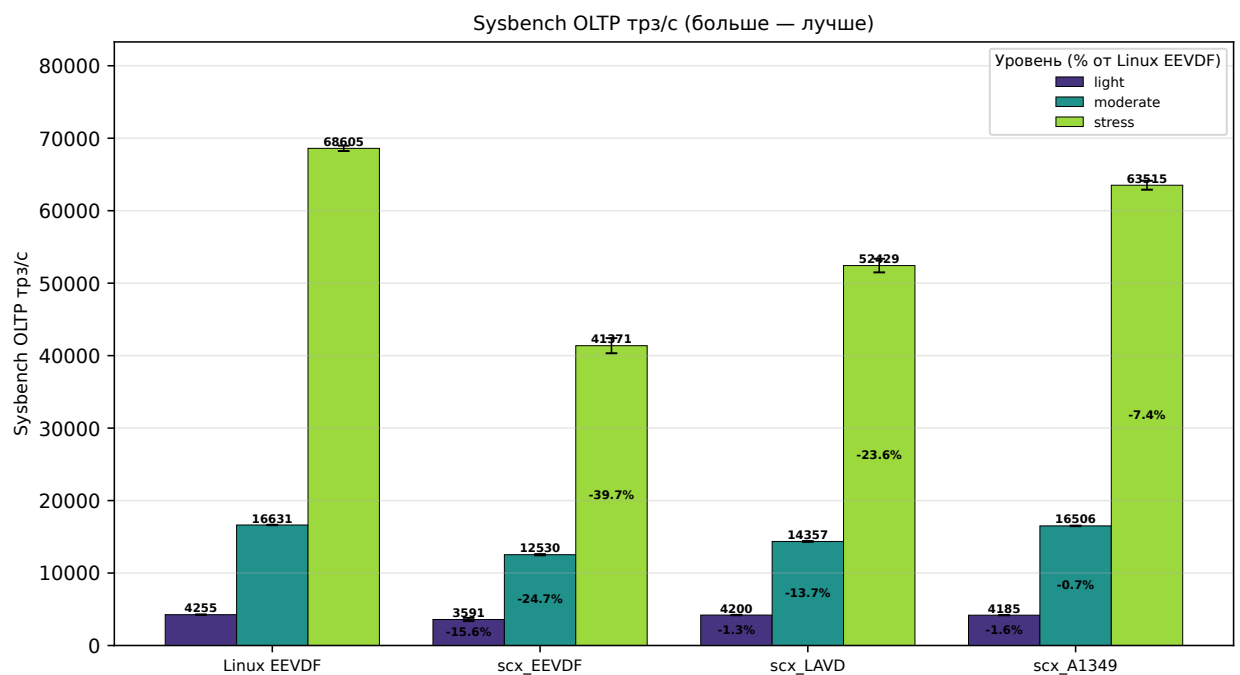
Рис. 5.4: Пропускная способность sysbench (TPS) для четырёх планировщиков по трём режимам нагрузки
