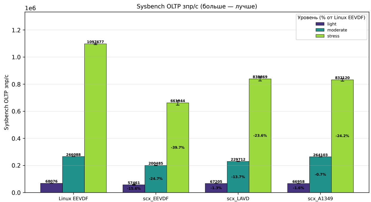
Рис. 5.5: Пропускная способность sysbench (QPS) для четырёх планировщиков по трём режимам нагрузки
