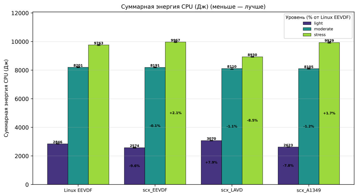
Рис. 5.12: Суммарное энергопотребление (Дж) для четырёх планировщиков по трём режимам нагрузки
