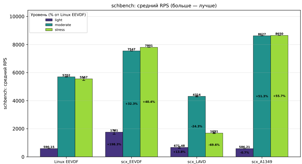
Рис. 5.6: Средняя пропускная способность schbench (запросов в секунду) для четырёх планировщиков по трём режимам нагрузки
