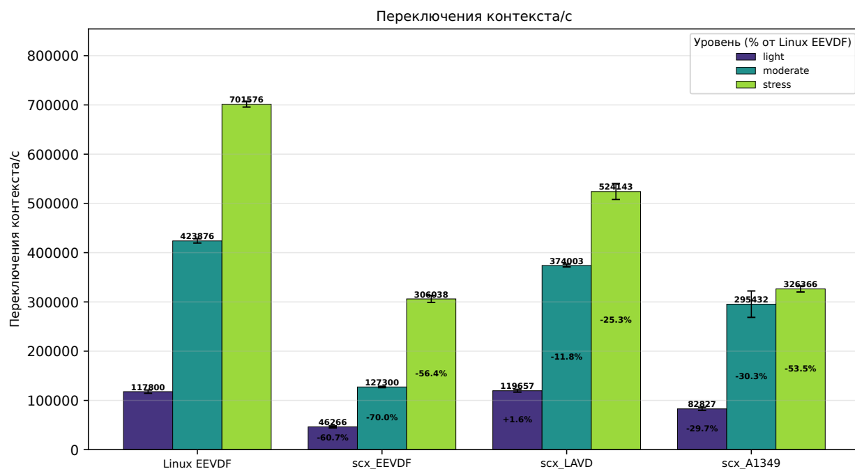
Рис. 5.10: Темп переключений контекста (число в секунду) для четырёх планировщиков по трём режимам нагрузки
