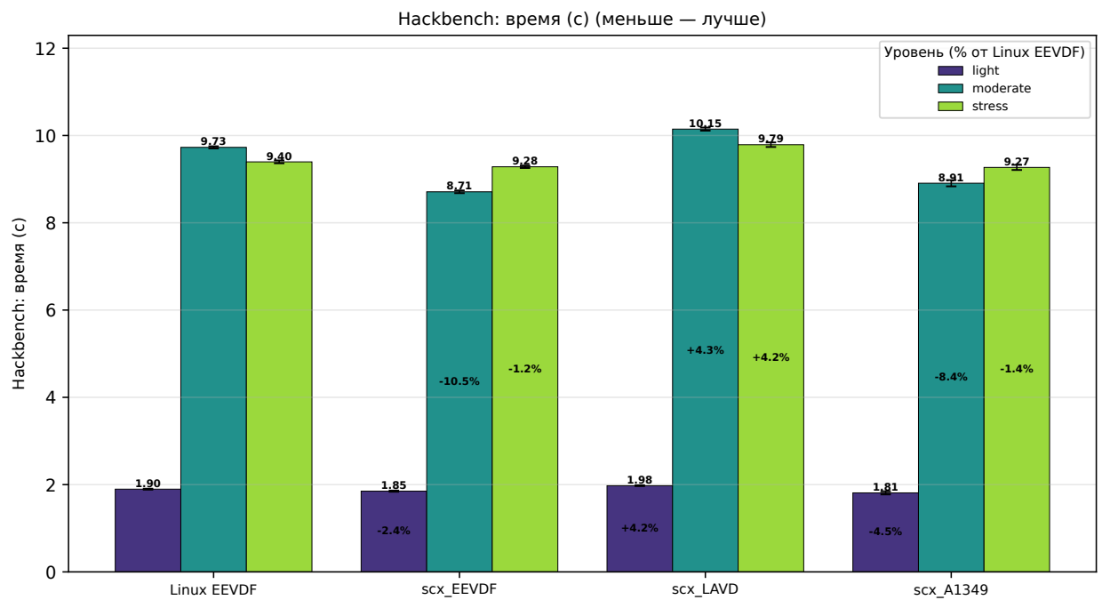
Рис. 5.3: Время выполнения hackbench (секунды) для четырёх планировщиков по трём режимам нагрузки
