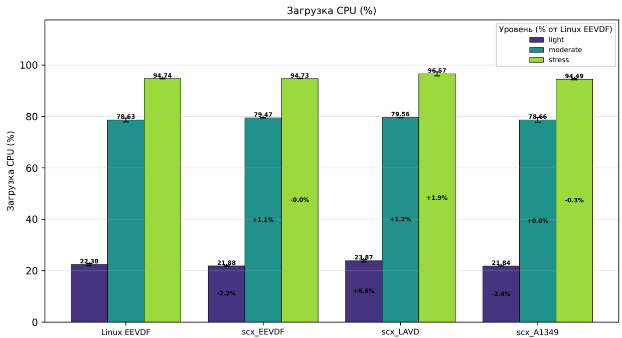
Рис. 5.11: Среднее использование CPU (%) для четырёх планировщиков по трём режимам нагрузки
