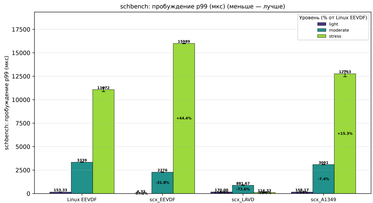
Рис. 5.7: Задержка пробуждения p99 schbench (мкс) для четырёх планировщиков по трём режимам нагрузки
