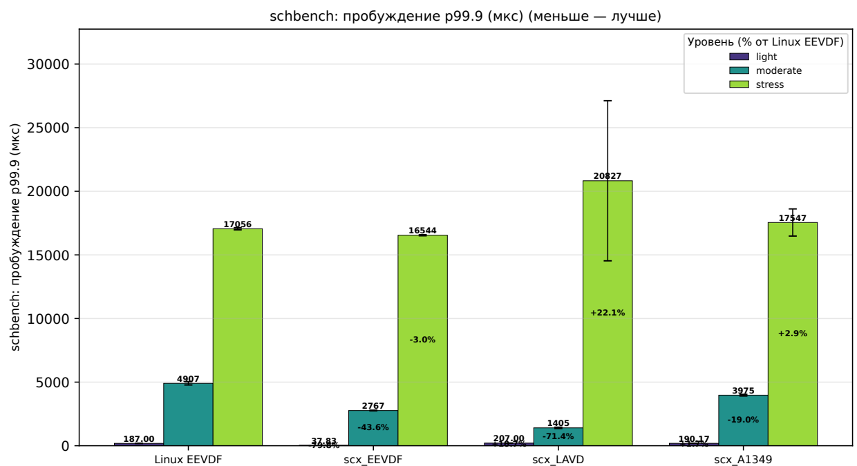
Рис. 5.8: Задержка пробуждения p99.9 schbench (мкс) для четырёх планировщиков по трём режимам нагрузки
