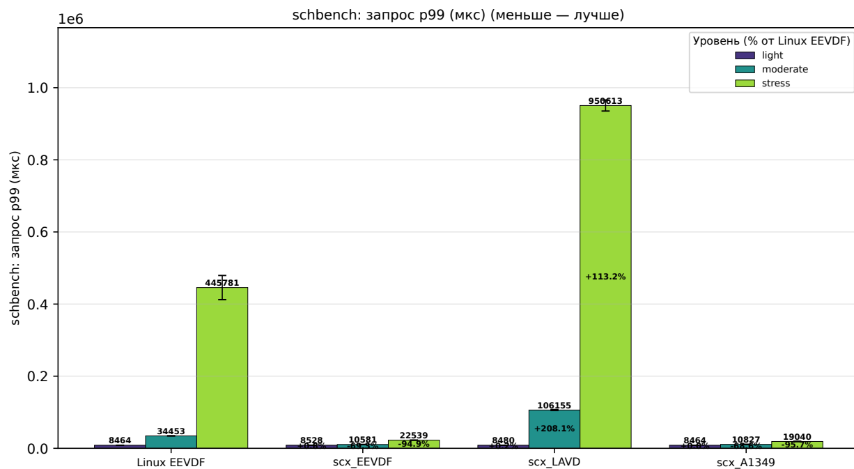
Рис. 5.9: Задержка запроса p99 schbench (мкс) для четырёх планировщиков по трём режимам нагрузки
