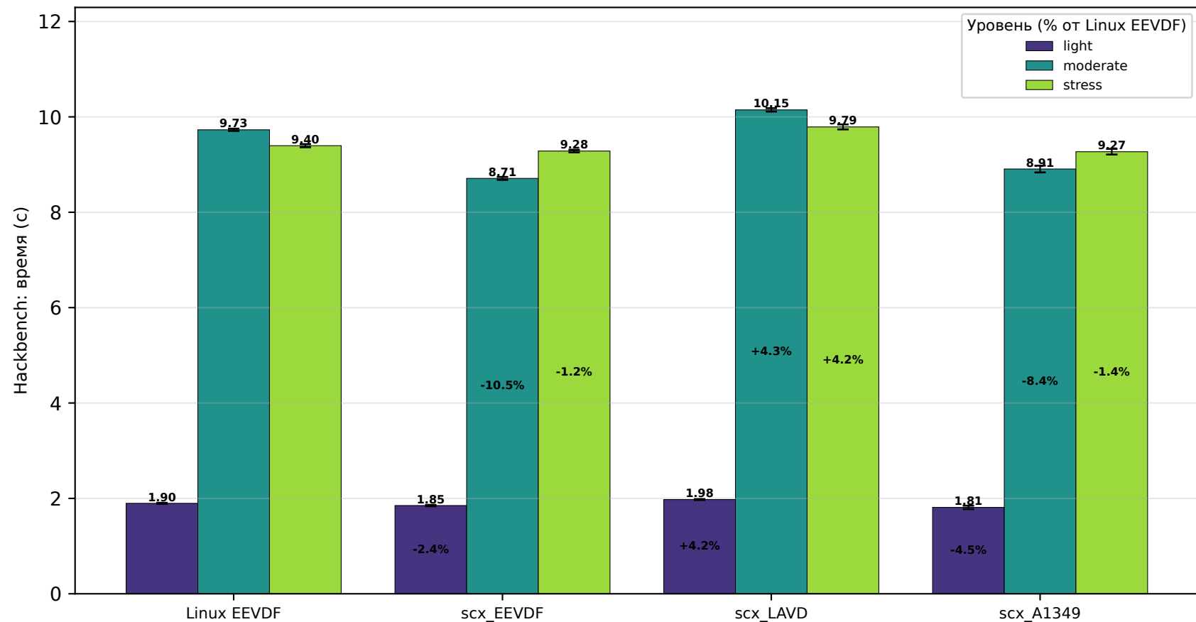
Наскбенч: время (с) (меньше — лучше)
