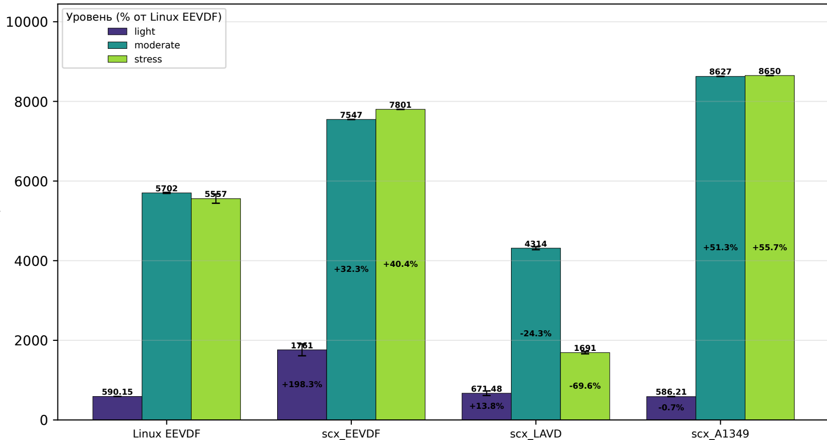
schbench: средний RPS (больше — лучше)
