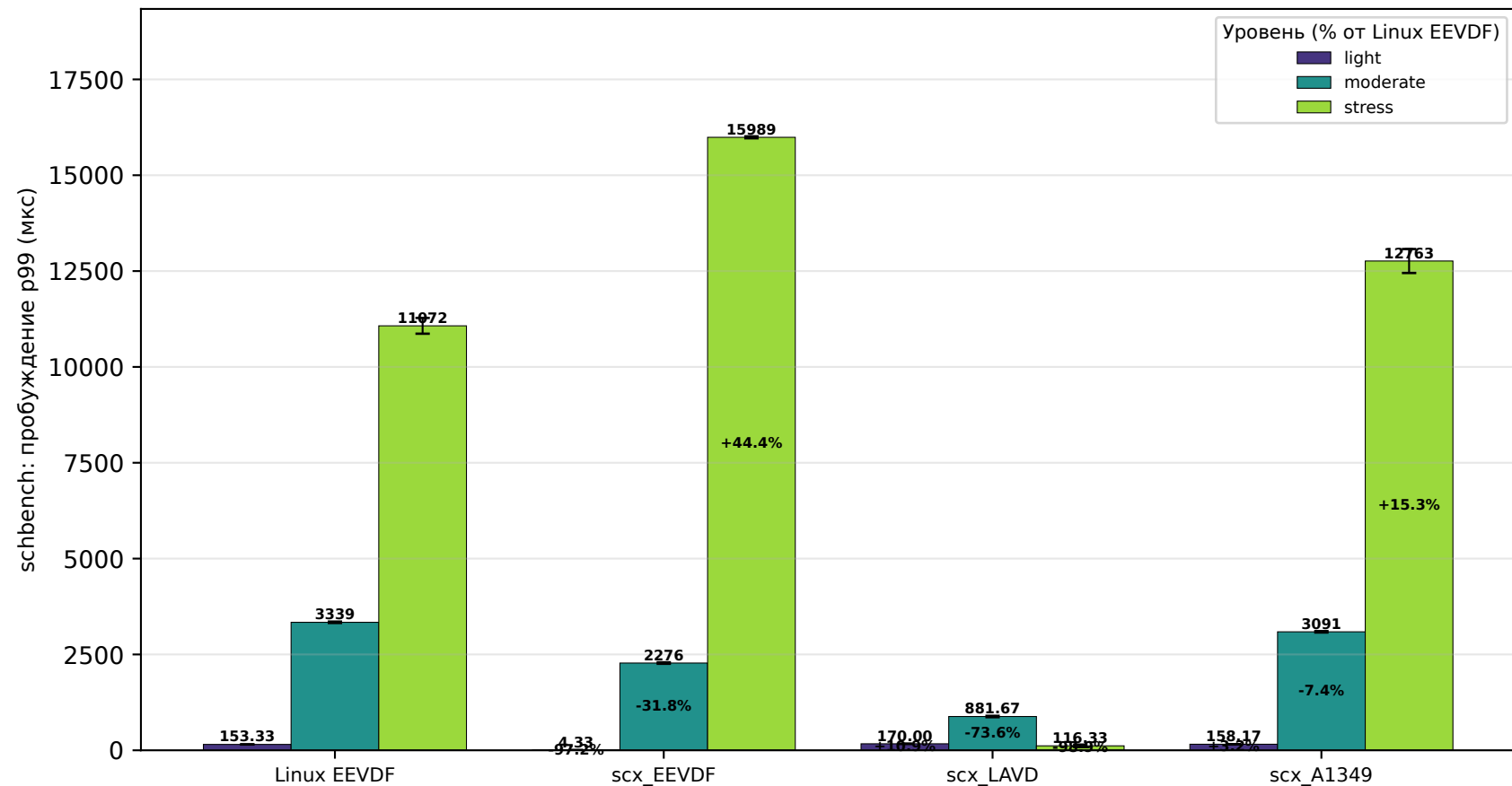
schbench: пробуждение p99 (мкс) (меньше — лучше)
