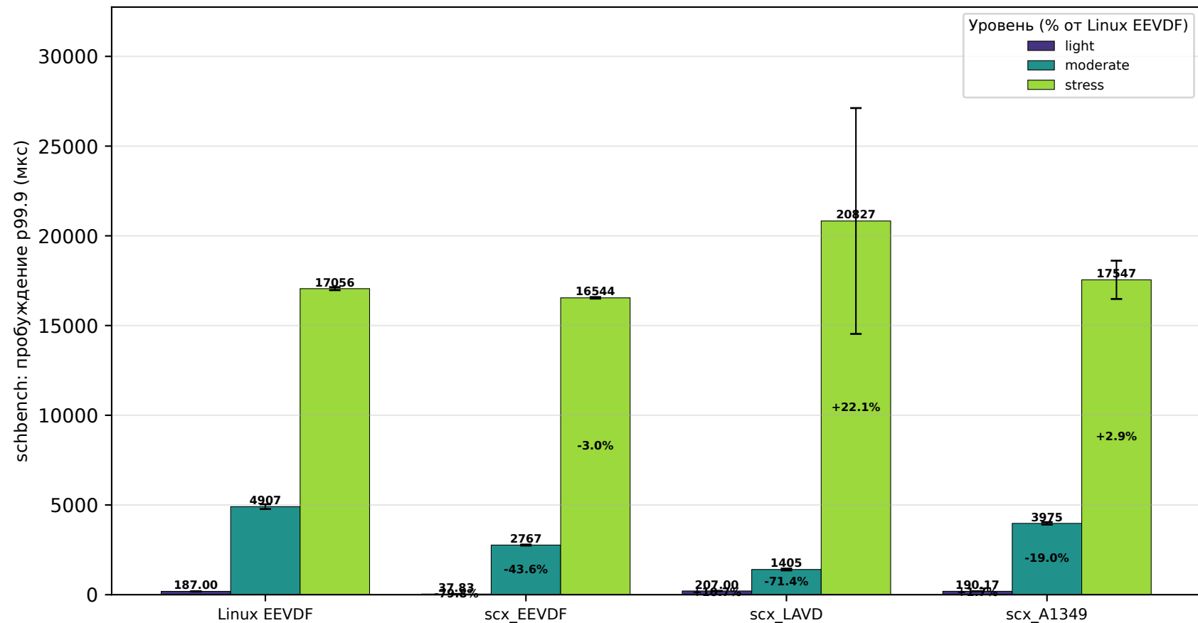
schbench: пробуждение p99.9 (мкс) (меньше — лучше)
