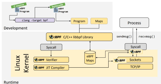
Рис. 1. eBPF в сетевой подсистеме
