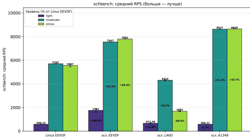
Рис. 4. Schbench: RPS
