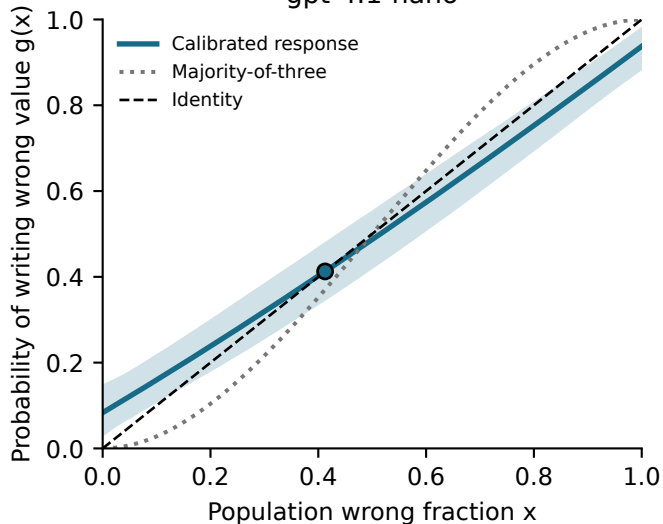
gpt-4.1-nano
