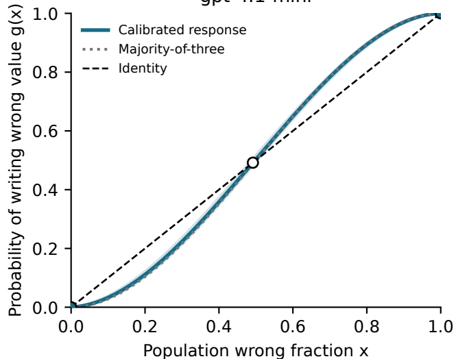
gpt-4.1-mini
