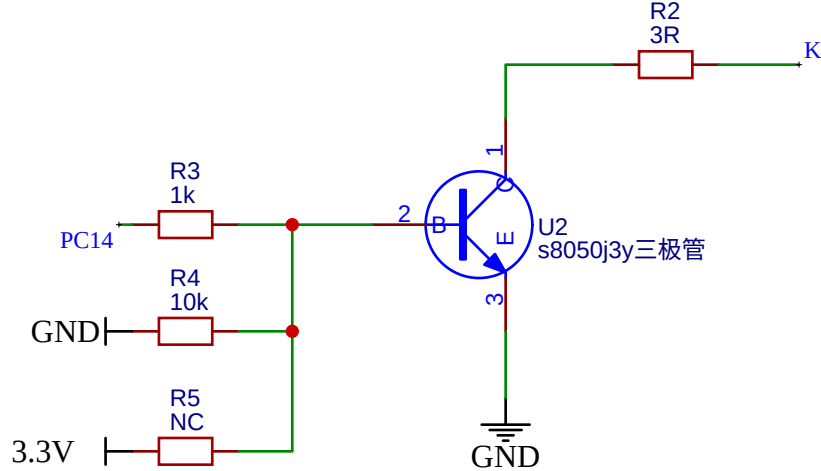
LCD背光控制电路
