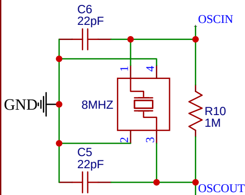
晶振电路
