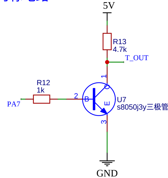
时标电路
