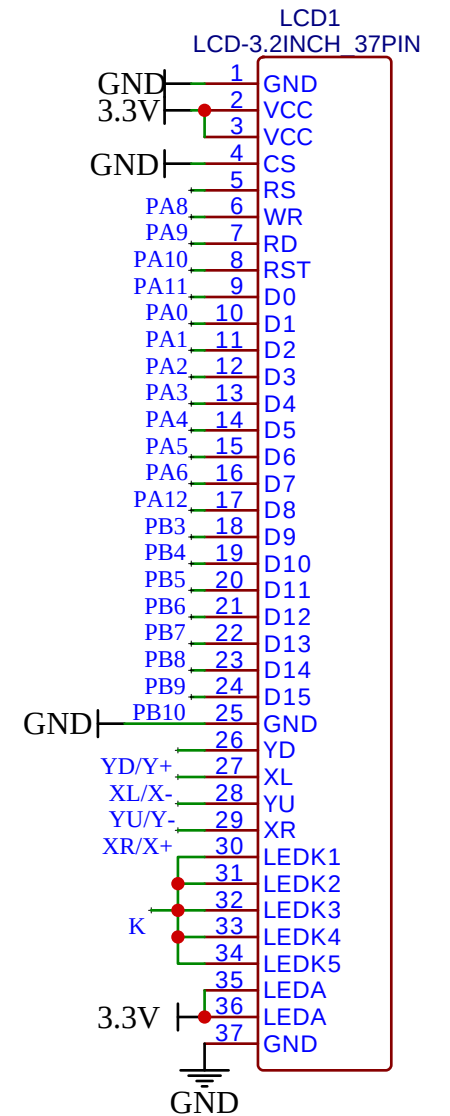
LCD显示屏
