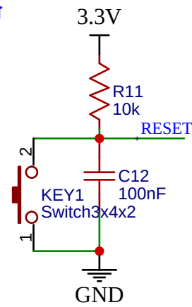
复位电路
