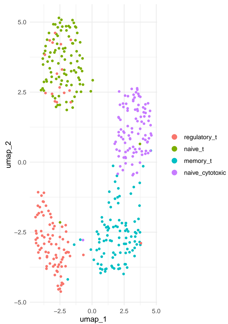
UMAP — true labels
