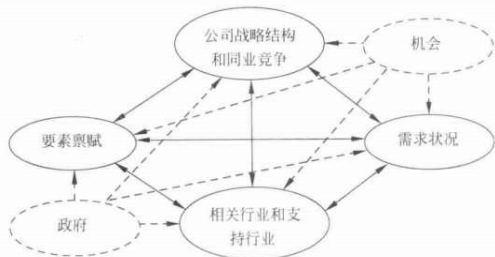
图 9-13 钻石模型
