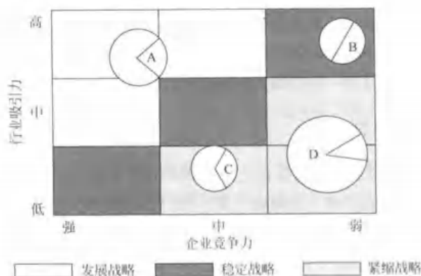
图 9-7 GE 矩阵
