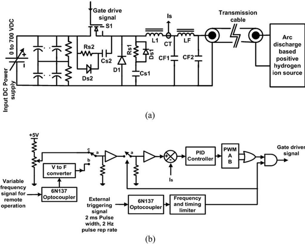
图 1.9.1: (a)CCPPS 功率电路, (b)CCPPS 控制电路。
