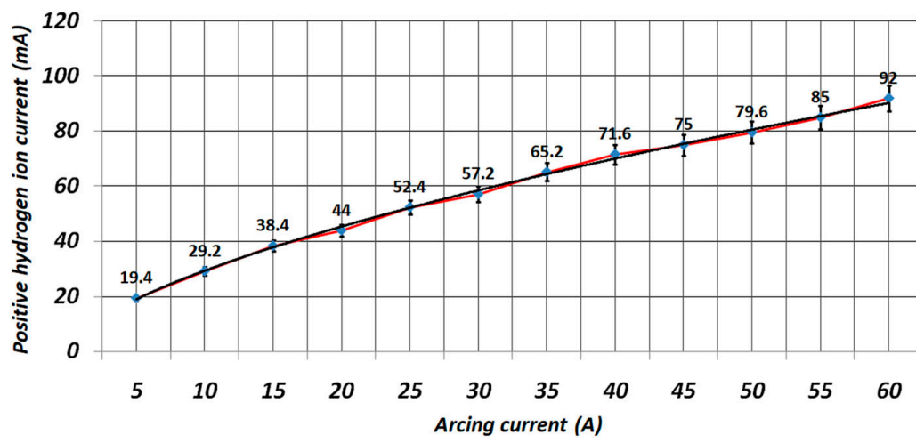
图 1.9.3: 引出质子电流与弧电流关系。
