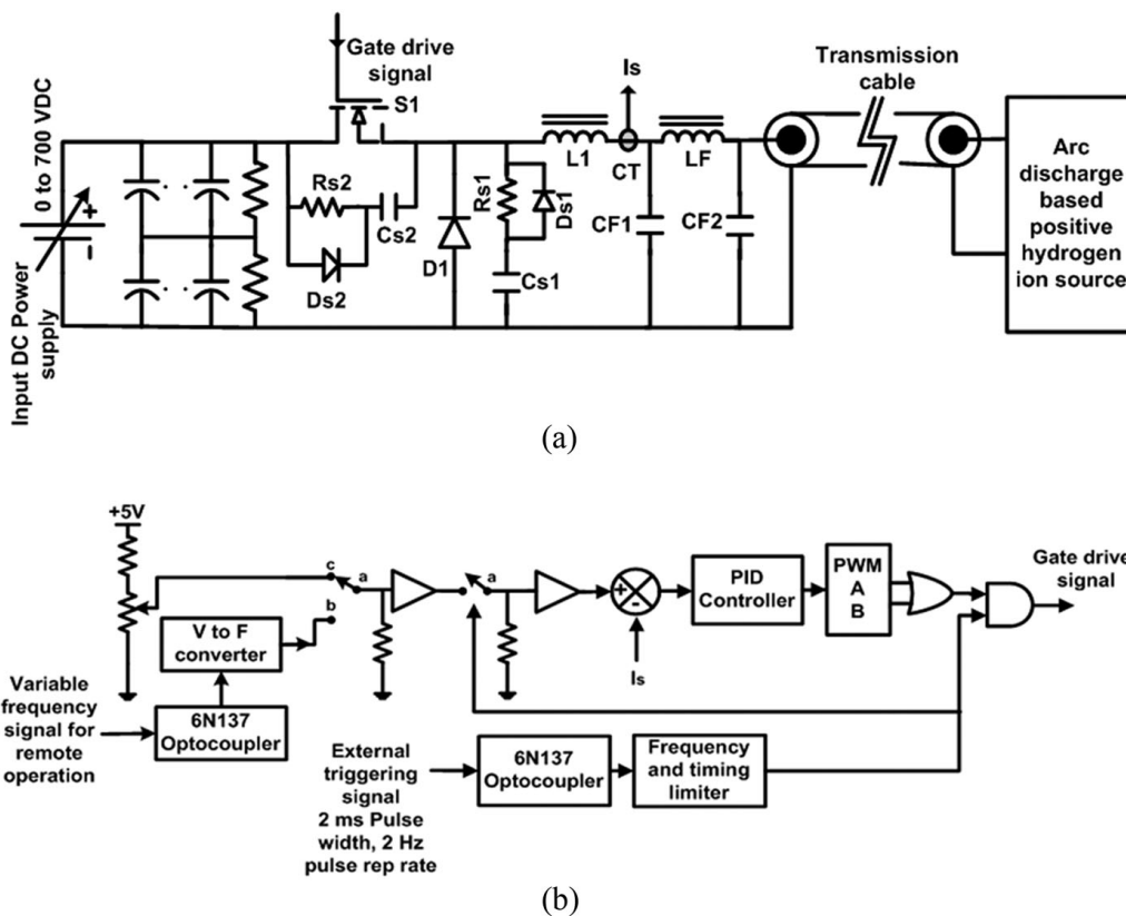
图 1.10.1: (a)CCPPS 功率电路, (b)CCPPS 控制电路。
