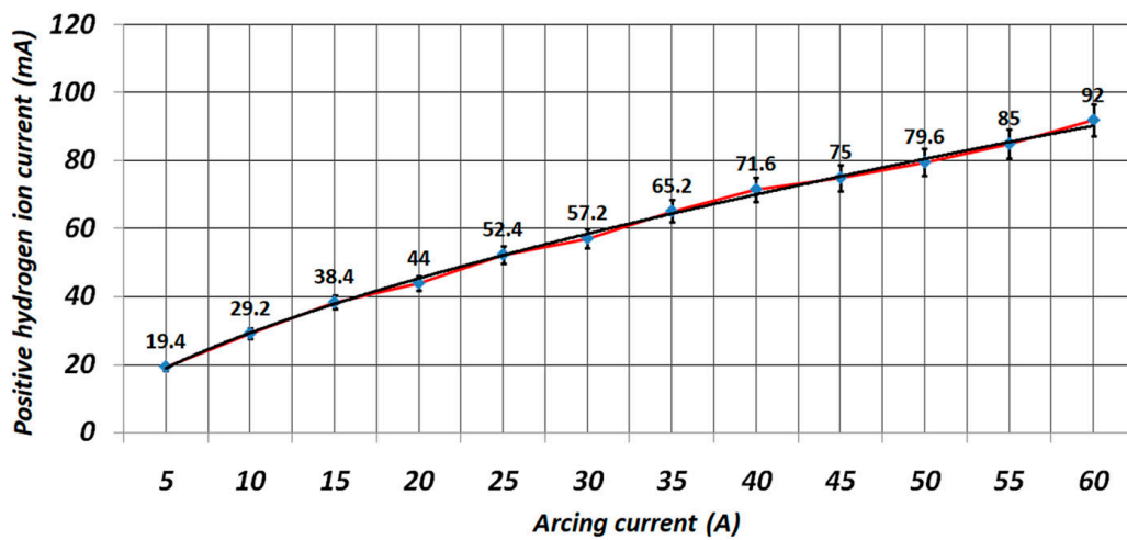
图 1.10.3: 引出质子电流与弧电流关系。
