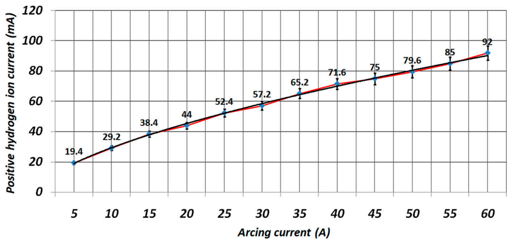
图 1.10.3: 引出质子电流与弧电流关系。
