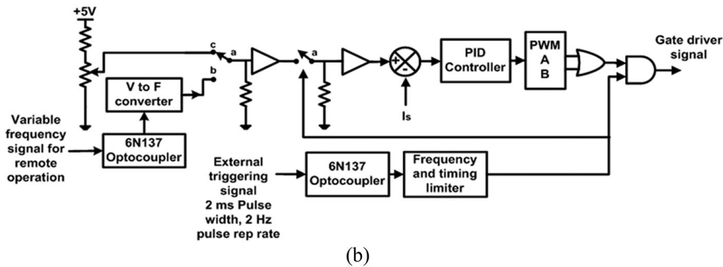
图 1.14.1: (a)CCPPS 功率电路，(b)CCPPS 控制电路。
