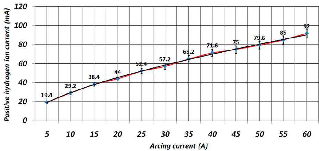
图 1.14.3: 引出质子电流与弧电流关系。
