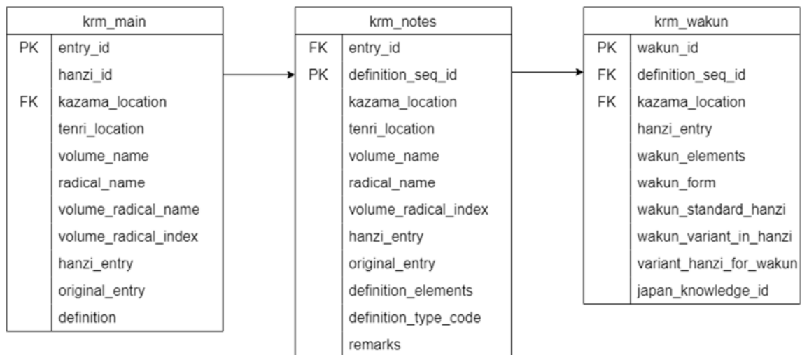
ER diagram.
