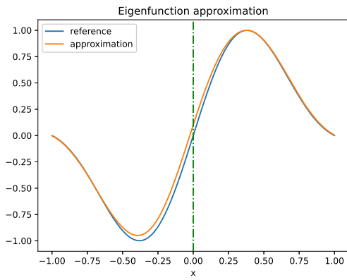
(e) 单位球上的第三特征函数 \hat{\xi}_{\phi 3}
