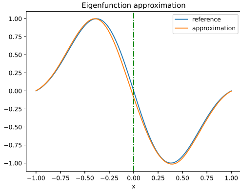
(c) 单位球上的第二特征函数 \hat{\xi}_{\phi 2}
