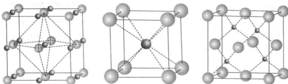
图 11: 三种典型的 AB 型离子晶体结构 (从左至右: NaCl 型、CsCl 型、立方 ZnS 型)
