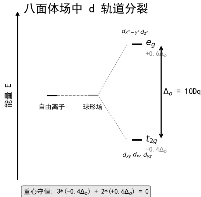
图 3: 八面体场中 d 轨道分裂
