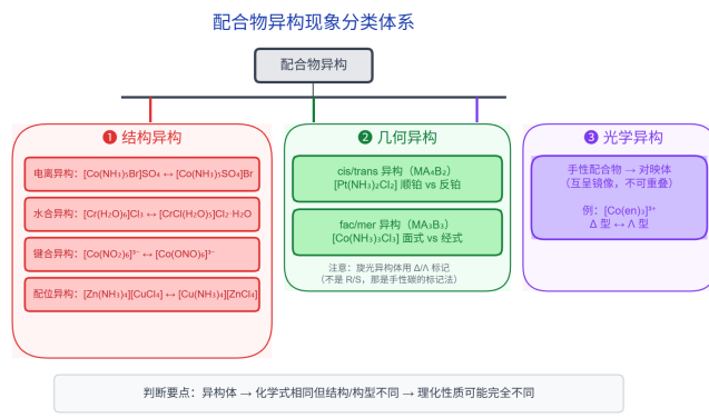
图 13: 配合物异构现象分类体系
