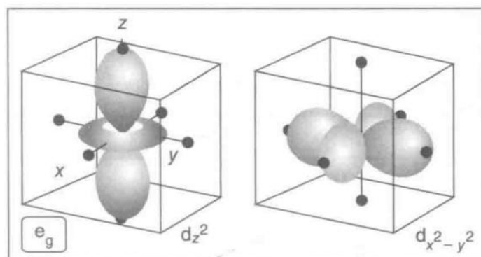
图 2: 八面体场中 e_g 轨道 ( d_{z^2} 和 d_{x^2-y^2} ) 的空间取向
