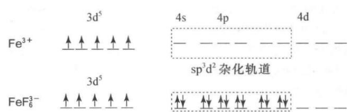
图 14: Fe 外轨型 (sp 3 d 2 ) 与内轨型 (d 2 sp 3 ) 杂化轨道对比
