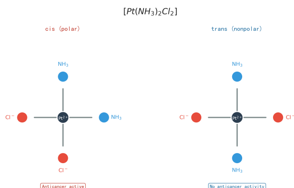
图 15: a [\text{Pt}(\text{NH})\text{Cl}] 顺式/反式几何异构体—顺铂有抗癌活性，反式无活性
