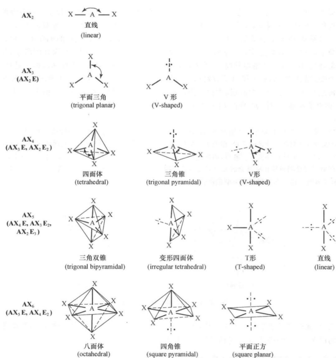
图 8: VSEPR 常见构型汇总 (AX-AX)
