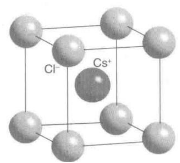
图 27: CsCl 型结构
