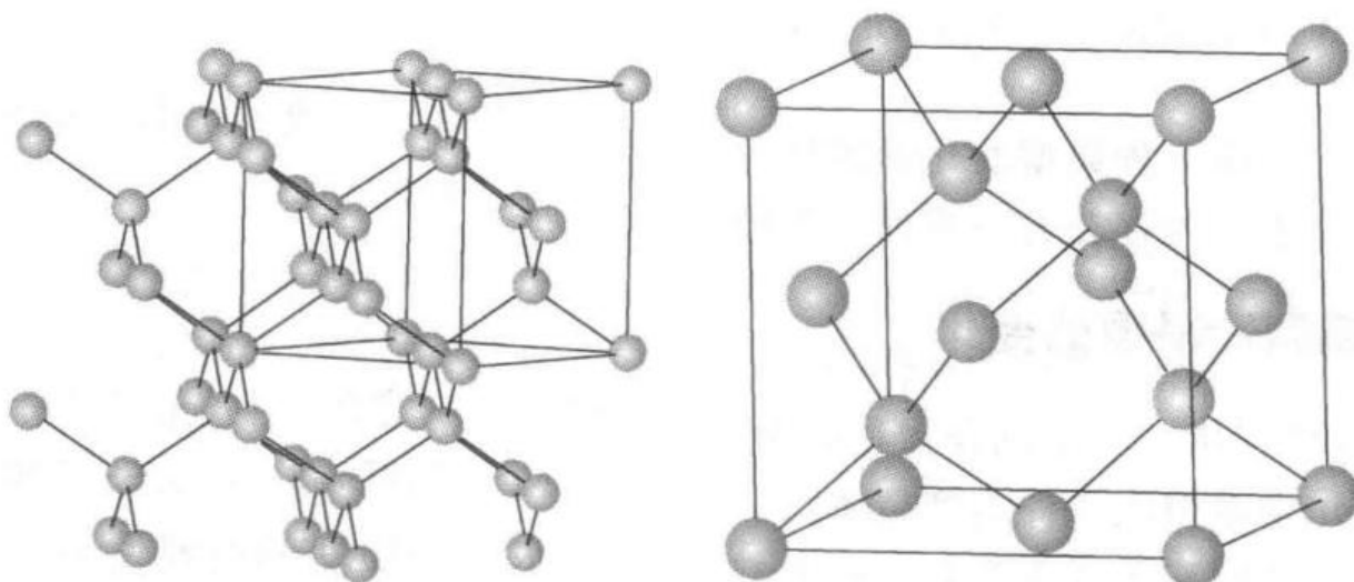
图 10: 金刚石的晶体结构与面心立方晶胞
