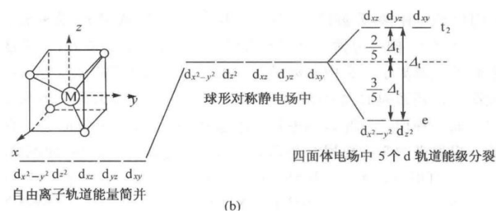
图 4: 四面体场中 d 轨道分裂
