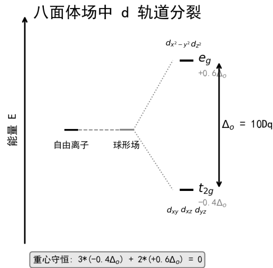
图 3: 八面体场中 d 轨道分裂
