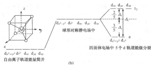
图 4: 四面体场中 d 轨道分裂
