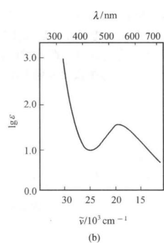
图 12: [Ti(HO)] 的 d-d 跃迁吸收光谱
