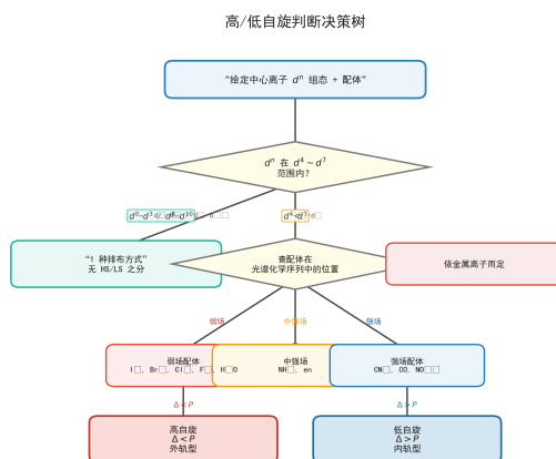
图 9: 高/低自旋判断决策树
