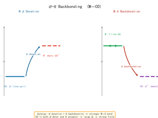
图 6: \sigma -反馈键示意图—CO 既是给体 (C 孤对电子), 又是受体 (M d 电子 *), 协同增强 M—C 键
