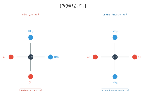
图 15: a [Pt(NH_3)_2Cl_2] 顺式/反式几何异构体—顺铂有抗癌活性, 反式无活性
