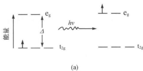
图 11: d-d 跃迁示意图
