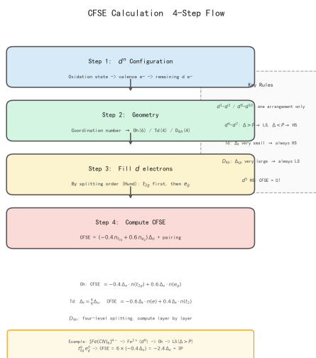
图 10: CFSE 计算四步流程
