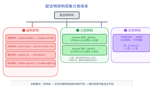
图 13: 配合物异构现象分类体系
