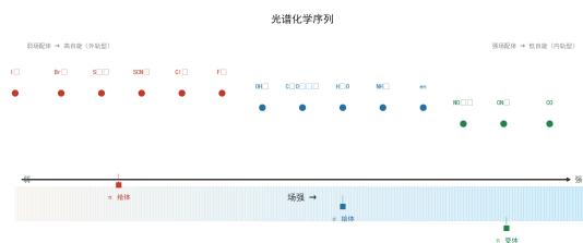
图 7: 光谱化学序列 (按场强排列, //)
