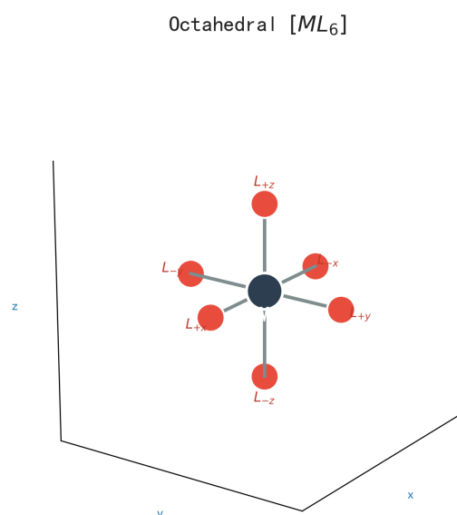
图 1: a 八面体配位立体图—6 个配体沿 \pm x 、 \pm y 、 \pm z 轴方向与中心金属 M 配位
