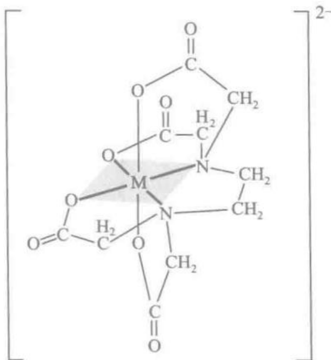
图 1: 图 EDTA 与中心金属 M 的八面体螯合结构
