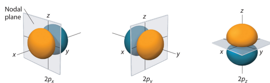
图 4: p 轨道的三种空间取向示意。
