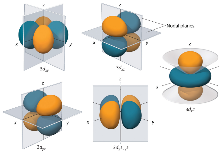
图 5: 五个 d 轨道的空间取向示意。
