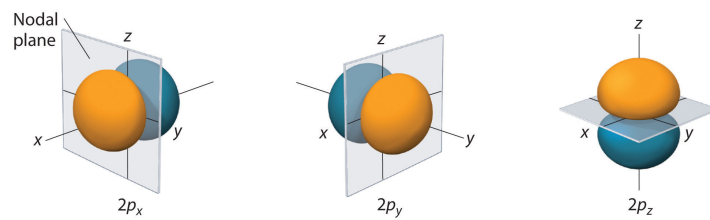
图 4: p 轨道的三种空间取向示意。
