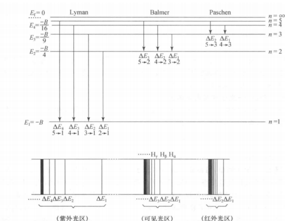
图 2 氢原子各系谱线形成示意图。 2. 玻尔三项革命性假设
