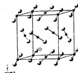
图 2 干冰的结构
