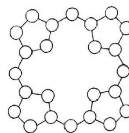
图 1 卟吩大环骨架
