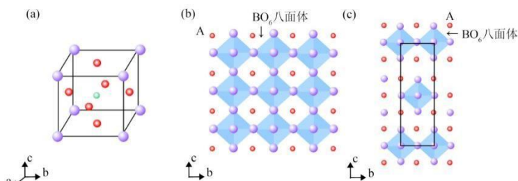
图 3 钙钛矿及其衍生结构
