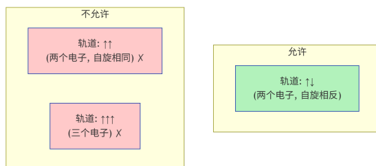
图 13: 图 14 Pauli 不相容原理示意图。
