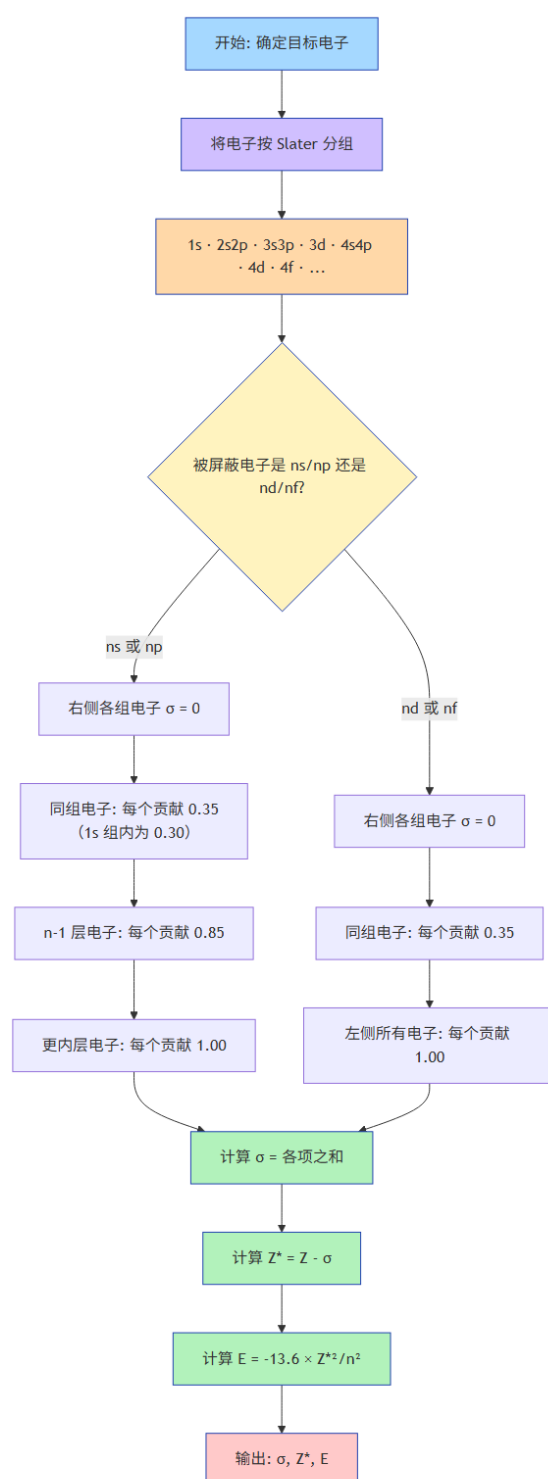
图 9: 图 10 Slater 规则计算流程图。
