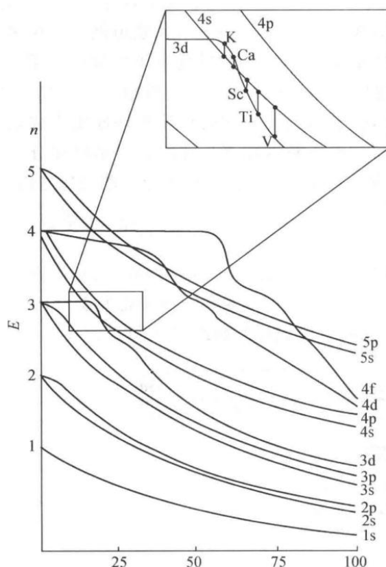
图 12: 图 13 Cotton 图，展示多电子原子轨道能量随原子序数 Z 的变化。
