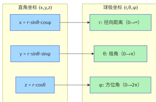
图 2: 图 3 直角坐标与球坐标的变量变换关系图。
