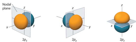
图 4: 图 5 p 轨道的三种空间取向示意。
