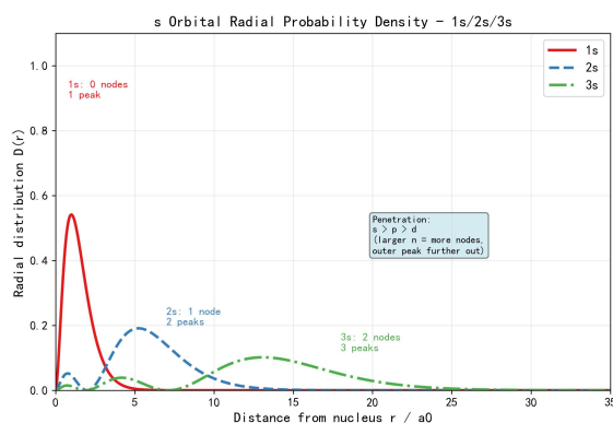
图 8: 图 9 1s、2s、3s 的径向概率密度分布。
