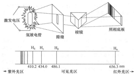
图 1: 图 1 可见光区的氢原子光谱。
