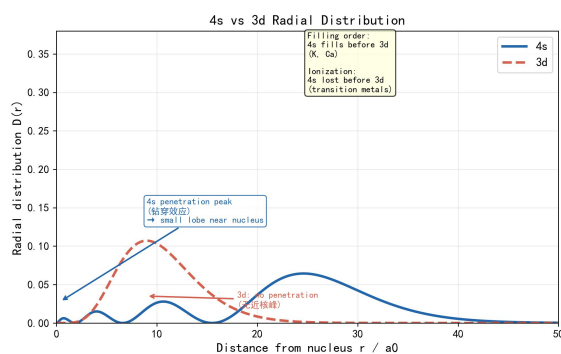
图 7: 图 8 4s 与 3d 的径向分布对比，展示 4s 的钻穿优势。
