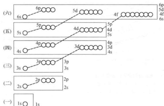
图 11: 图 12 Pauling 近似能级图。
