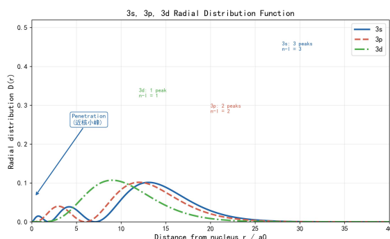
图 6: 图 7 3s、3p、3d 的径向分布函数对比，突出 s 轨道的近核小峰。
