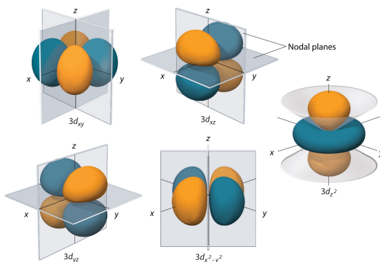
图 5: 图 6 五个 d 轨道的空间取向示意。
