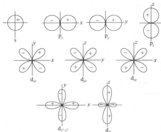
图 3: 图 4 s、p、d 轨道的角度分布示意。
