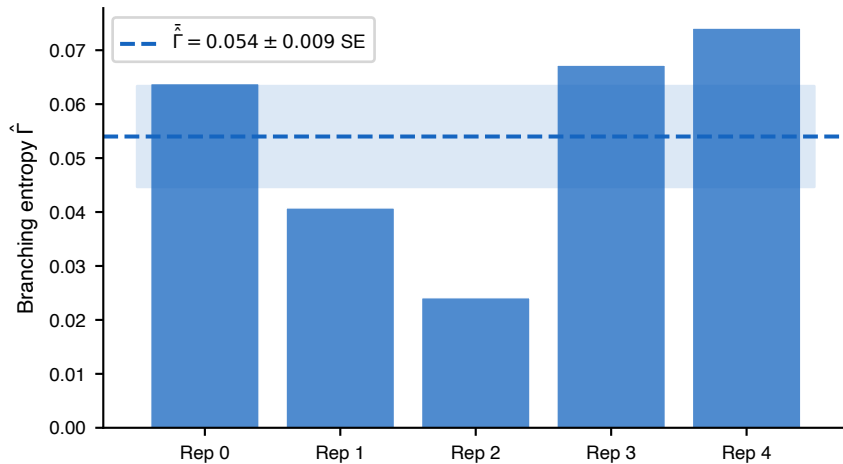
(A) \hat{\Gamma} per replicate (IM-01, T = 0.7 , K = 30 )
