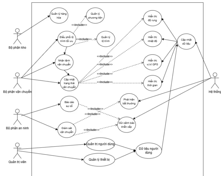
Hình 3.5.1: Usecase diagram
