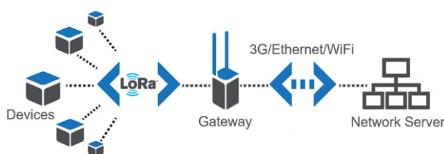
Hình 2.3.1: Minh họa về công nghệ LoRa
