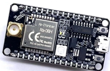
Hình 2.5.5: Module LoRa Ra-08H Development Board Ai-Thinker
