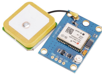
Hình 2.4.4: Module GPS NEO-6MV2
