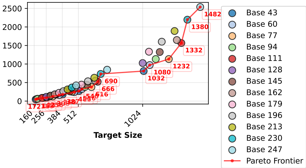
Total DSP Slices
