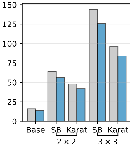
DSP Slices
