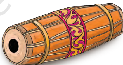
Fig. 7.4. Mṛidaṅgam
