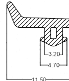
SMI-UPVC : 0003 Wt/mtr : 40 gm/mtr
