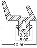
SMI-UPVC : 0001 Wt/mtr : 110 gm/mtr
