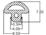
SMI-UPVC : 0008 Wt/mtr : 38 gm/mtr
