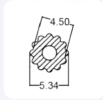
SMI-UPVC : 0018 Wt/mtr : 24 gm/mtr
