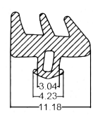
SMI-UPVC : 0012 Wt/mtr : 64 gm/mtr
