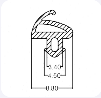
SMI-UPVC : 0017 Wt/mtr : 40 gm/mtr
