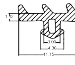
SMI-UPVC : 0015 Wt/mtr : 38 gm/mtr
