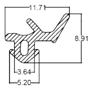
SMI-UPVC : 0005 Wt/mtr : 40 gm/mtr
