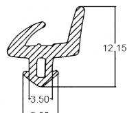
SMI-UPVC : 0010 Wt/mtr : 58 gm/mtr
