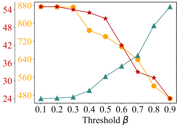
(a) PyTorch
