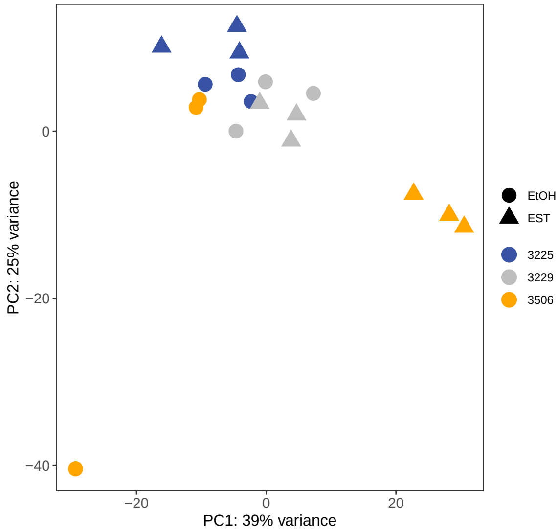
ChIP-seq PCA (All Samples)
