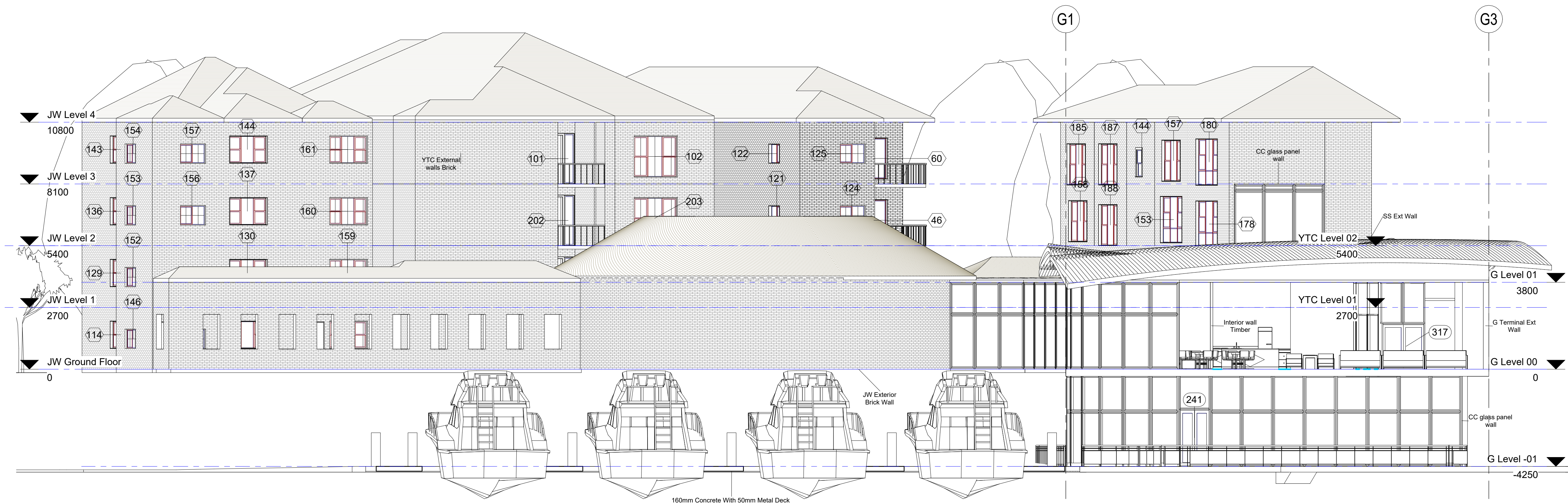
1 G Section 1 1 : 100
