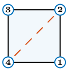
关于对角线 24 反射
