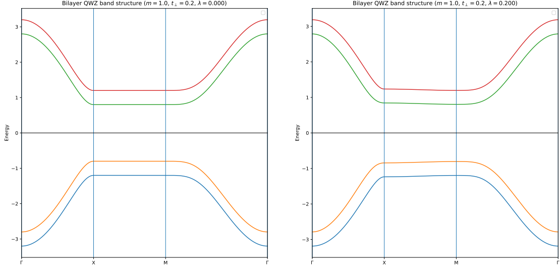
Figure 1: Bilayer QWZ 模型能带结构图，其中 \lambda 分别为 0 和 0.2
