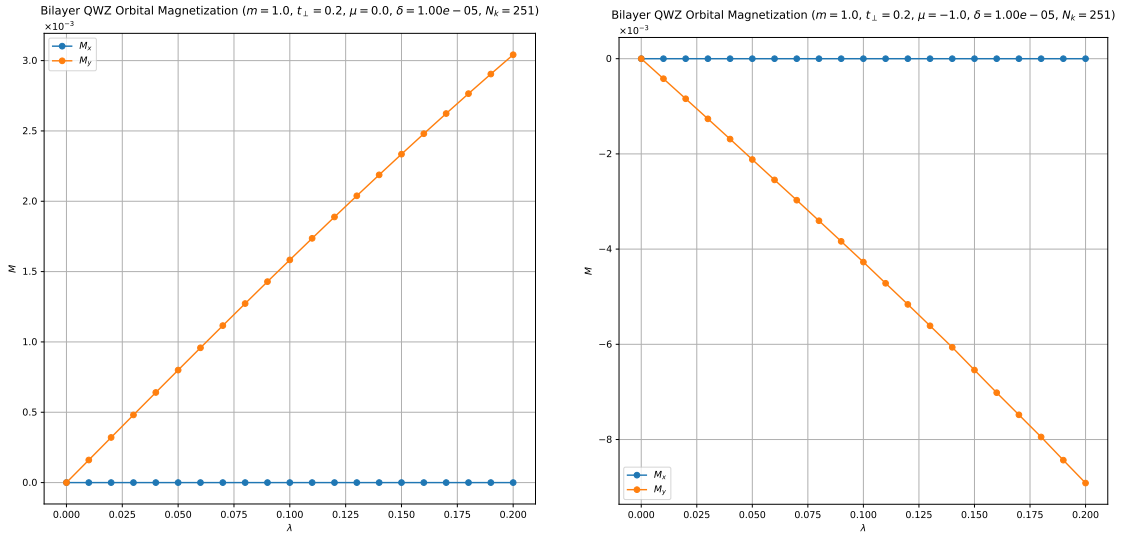
Figure 2: Bilayer QWZ 模型轨道磁化 M_y 示意图，其中化学势 \mu 分别取 0 和 -1
