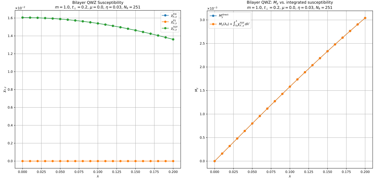
Figure 3: \mu = 0 时的 M_y 示意图
