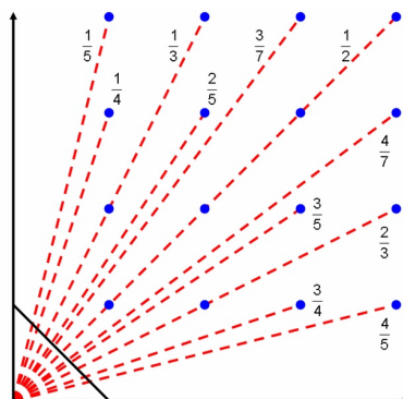
איור 4.16: הפרדס של אוקלידס
