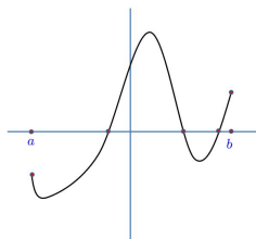
איור 4.19: ערך ביניים
