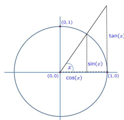
איור 4.6: מיהו טנגנס גאומטרית
