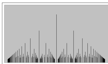
איור 4.17: הפרדס של אוקלידס בפרספקטיבה מהראשית
