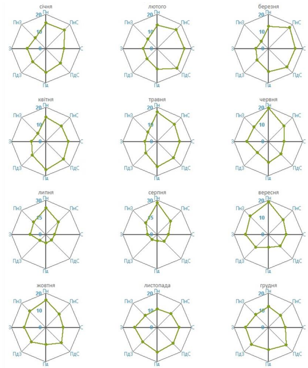
Рис.2.7. Повторюваність (%) напрямку вітру та штилю
