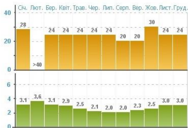
Рис.2.5. Середня місячна і максимальна кількість опадів (мм) з поправками на змочування
