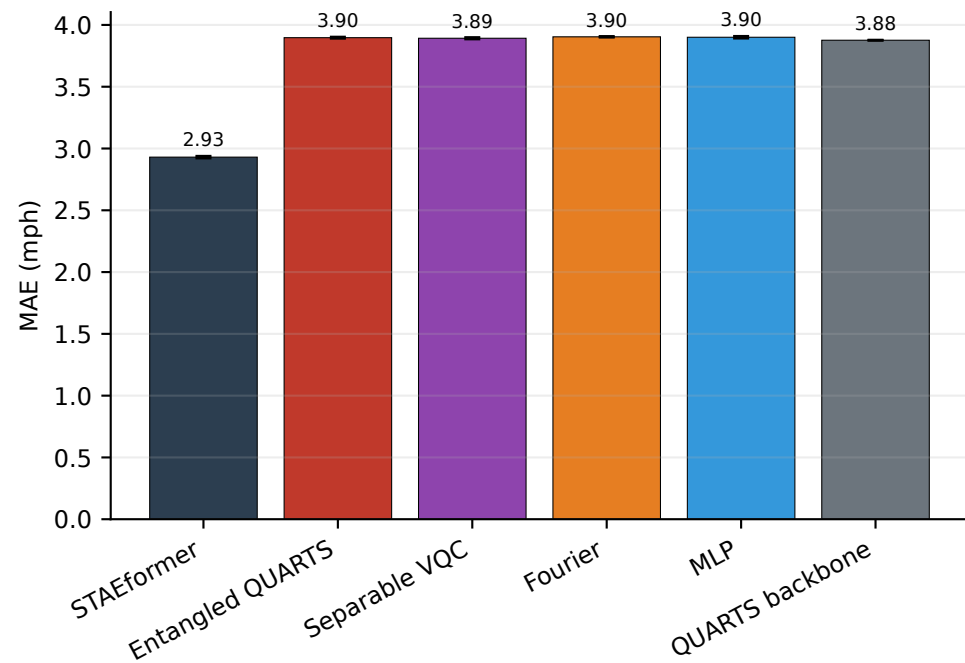
METR-LA
