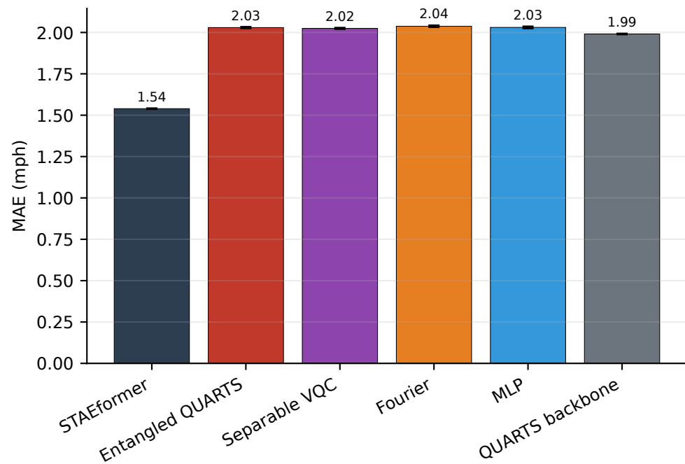
PEMS-BAY
